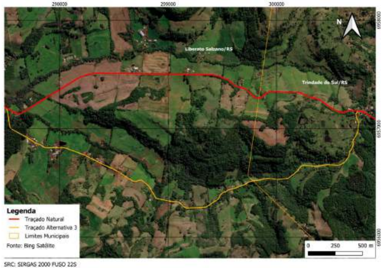
Figura 112 – Comparação entre Natural X Alternativa 03.
