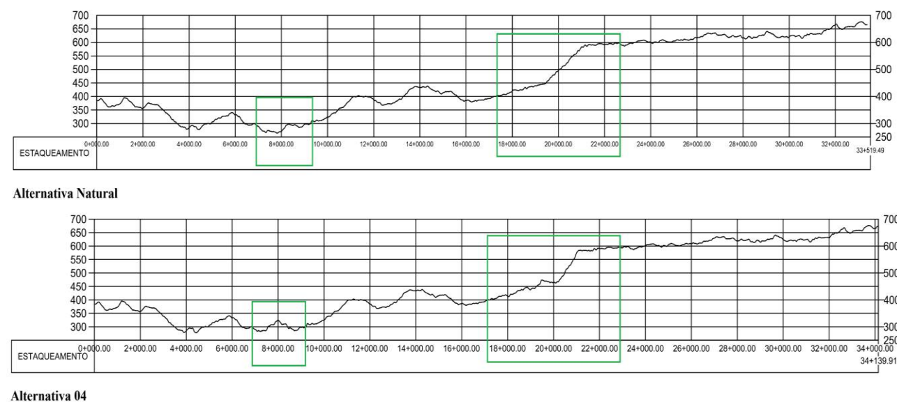
Figura 115 – Comparação entre perfis altimétricos (Natural X Alternativa 04).
