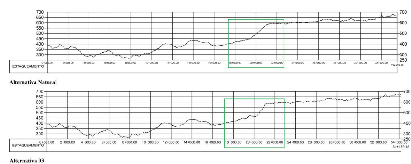
Figura 113 – Comparação entre perfis altimétricos (Natural X Alternativa 03).
